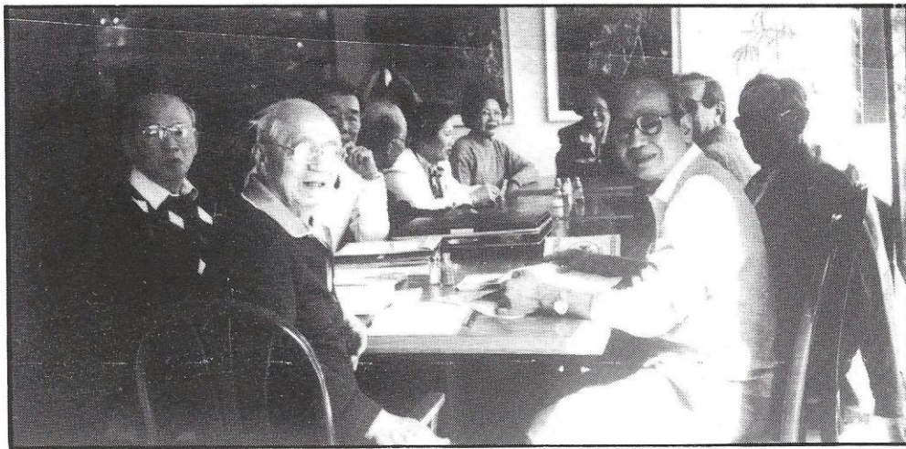
Liên-lạc số Đặc biệt TẾT phải tăng cường thêm nhân lực phái nữ để có thêm xăng nhớt (Từ trái qua : các Anh : Thoại, Tỉnh, Thường, Rạng và các Chị Thường, Vy, Tý, C. Cường (khuất), A. Cường, A. Thiết (đen mặt) và A. Thọ.
